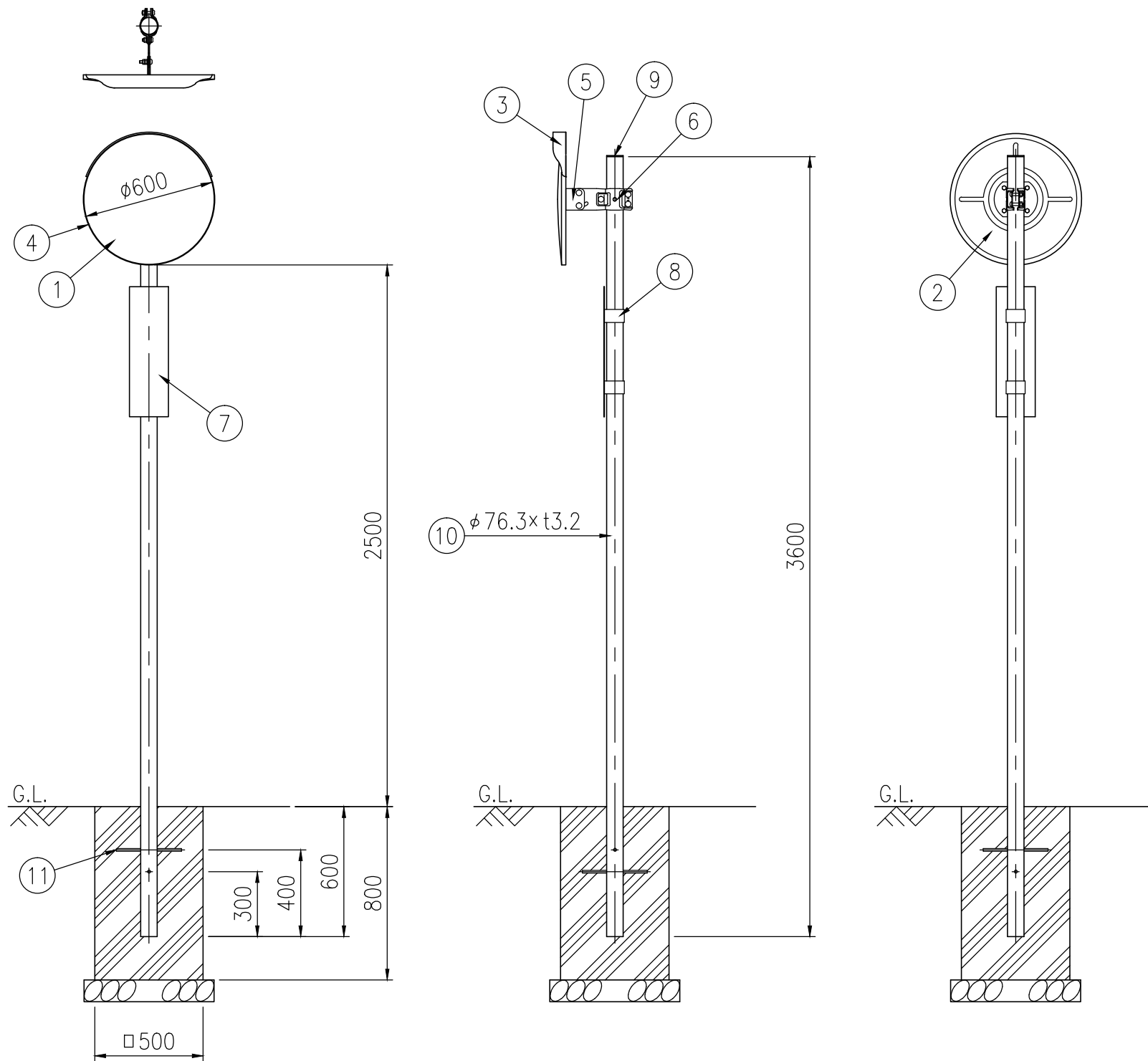
設置図 S=1/25
