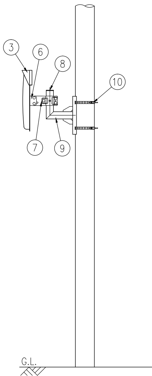
設置図 S=1/25
