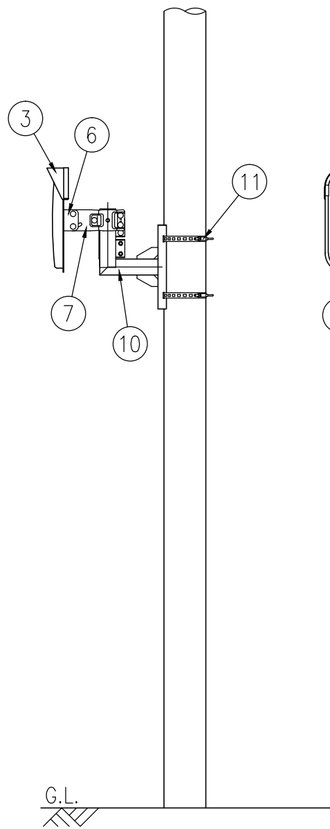
設置図 S=1/25
