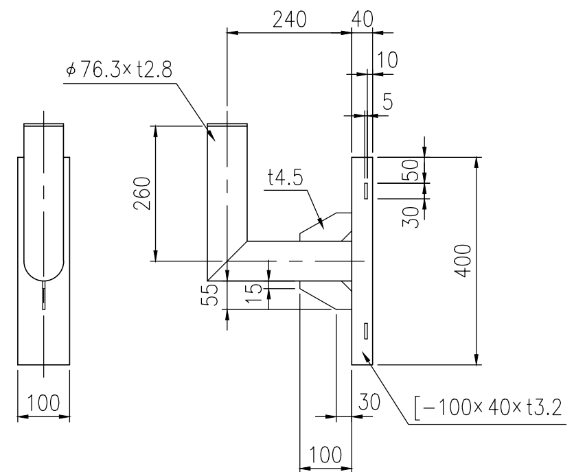
⑩ 電柱取付金具詳細図 S=1/10
