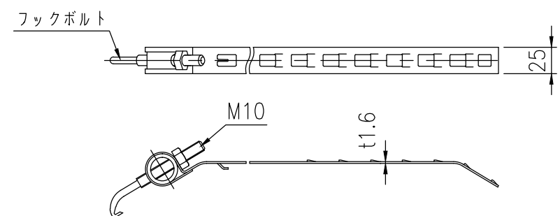
⑪ 取付バンド詳細図 S=1/5
