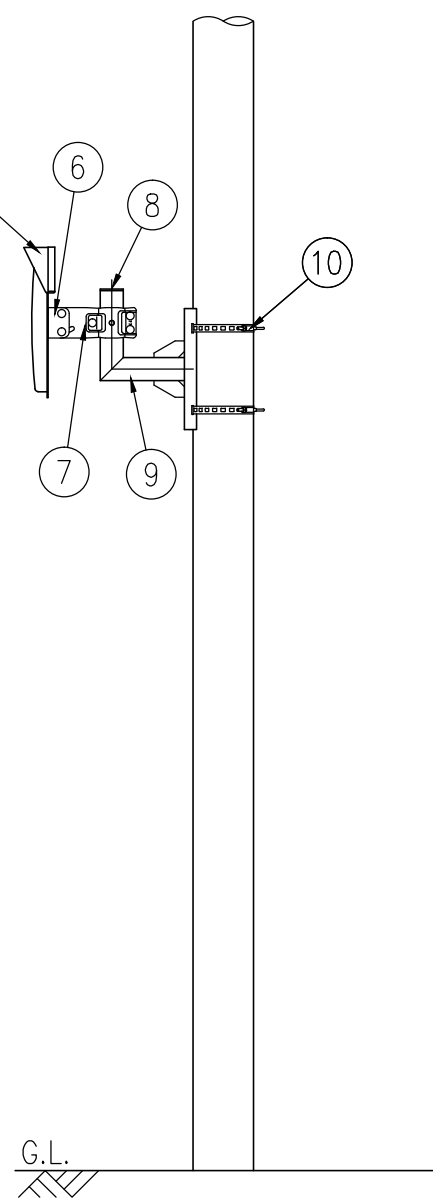
設置図 S=1/25
