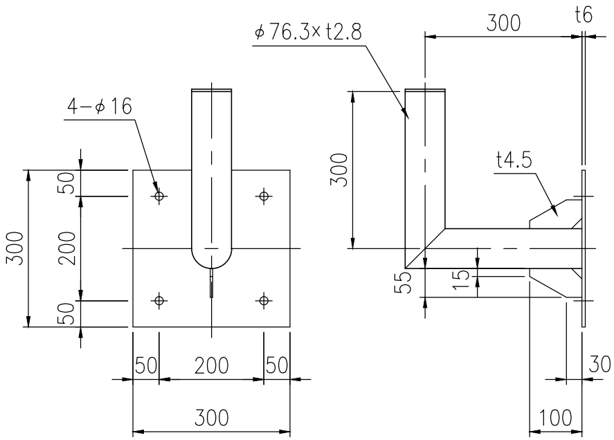
⑩よう壁取付金具詳細図 S=1/10
