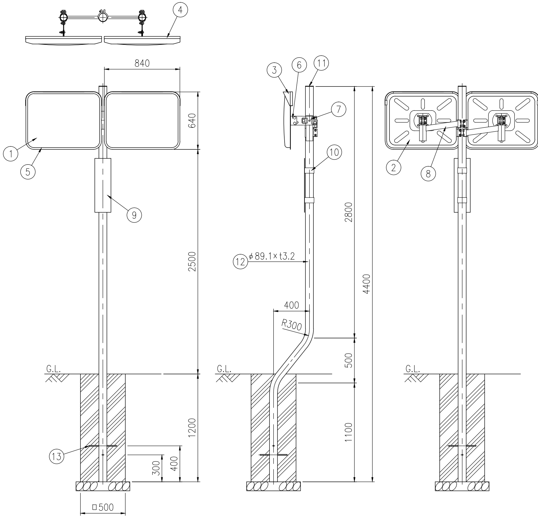
設置図 S=1/25
