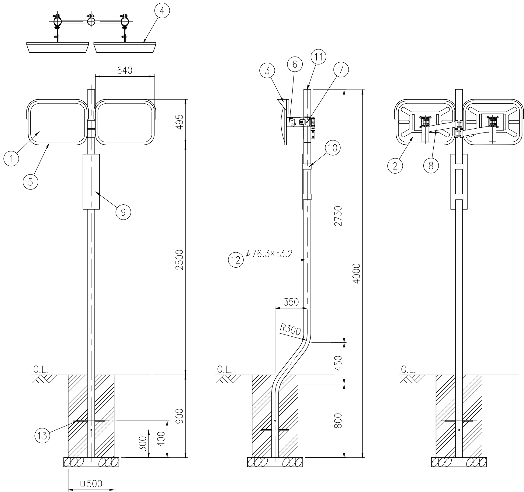
設置図 S=1/25
