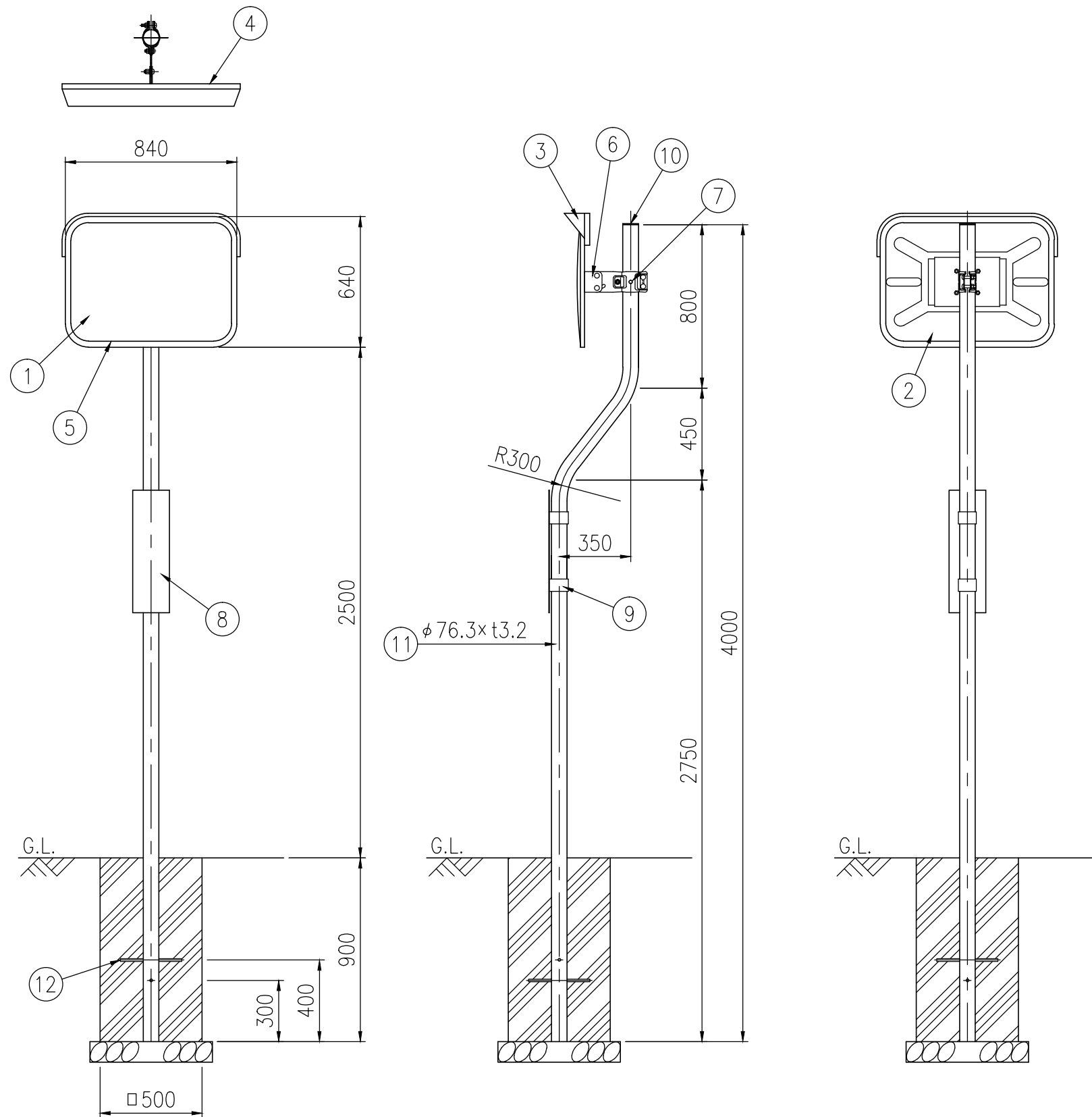
設置図 S=1/25
