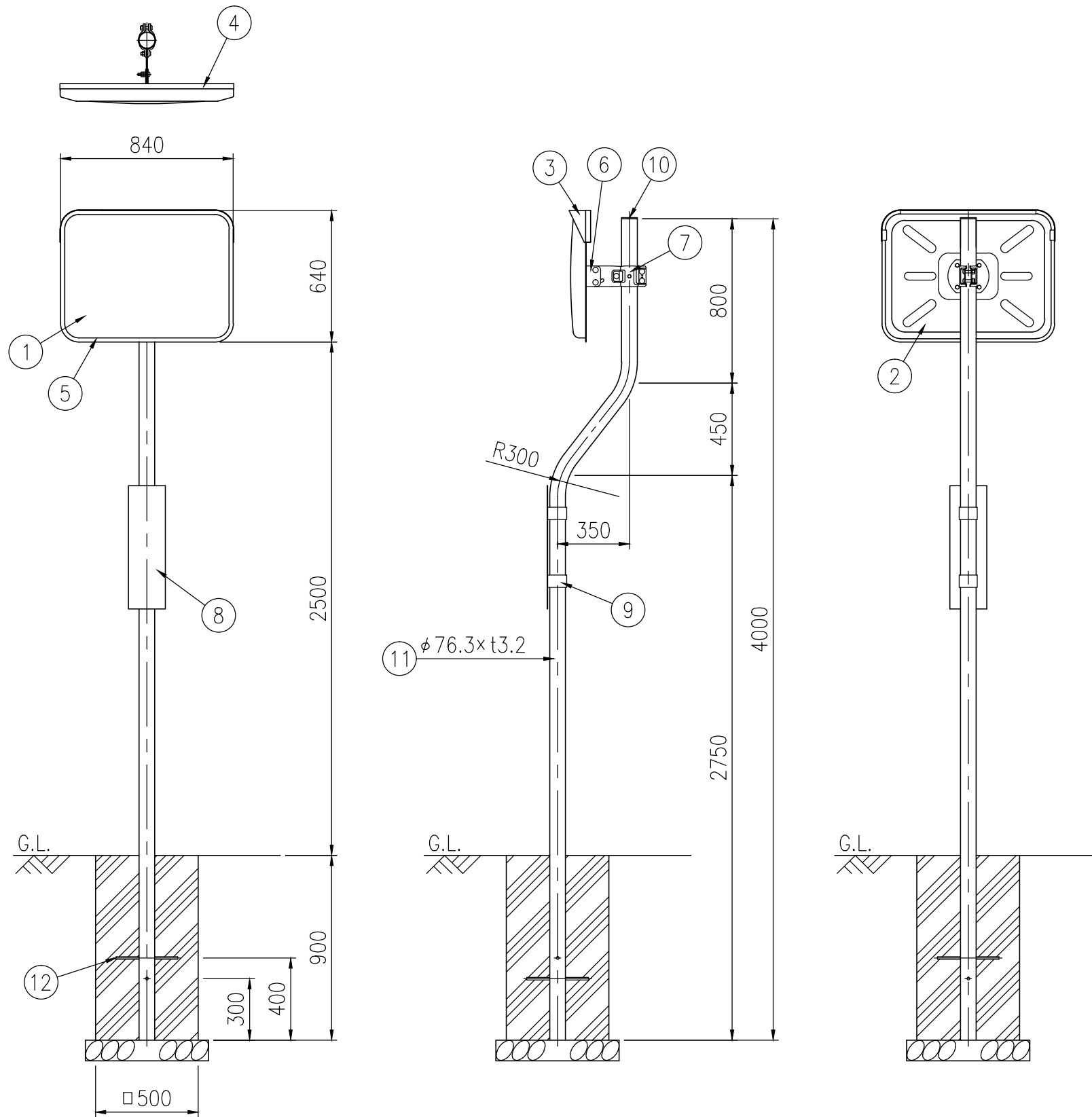
設置図 S=1/25
