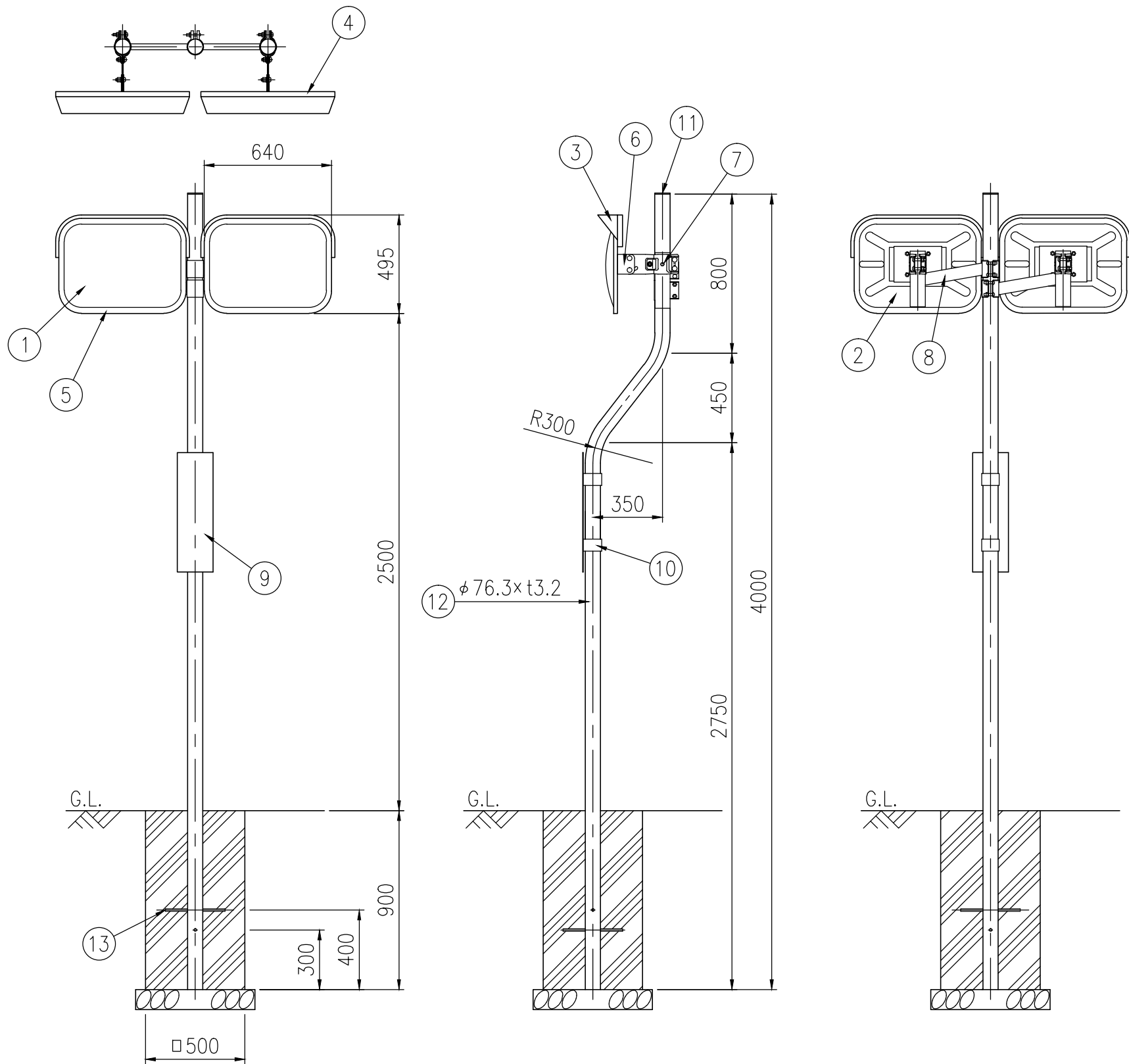
設置図 S=1/25
