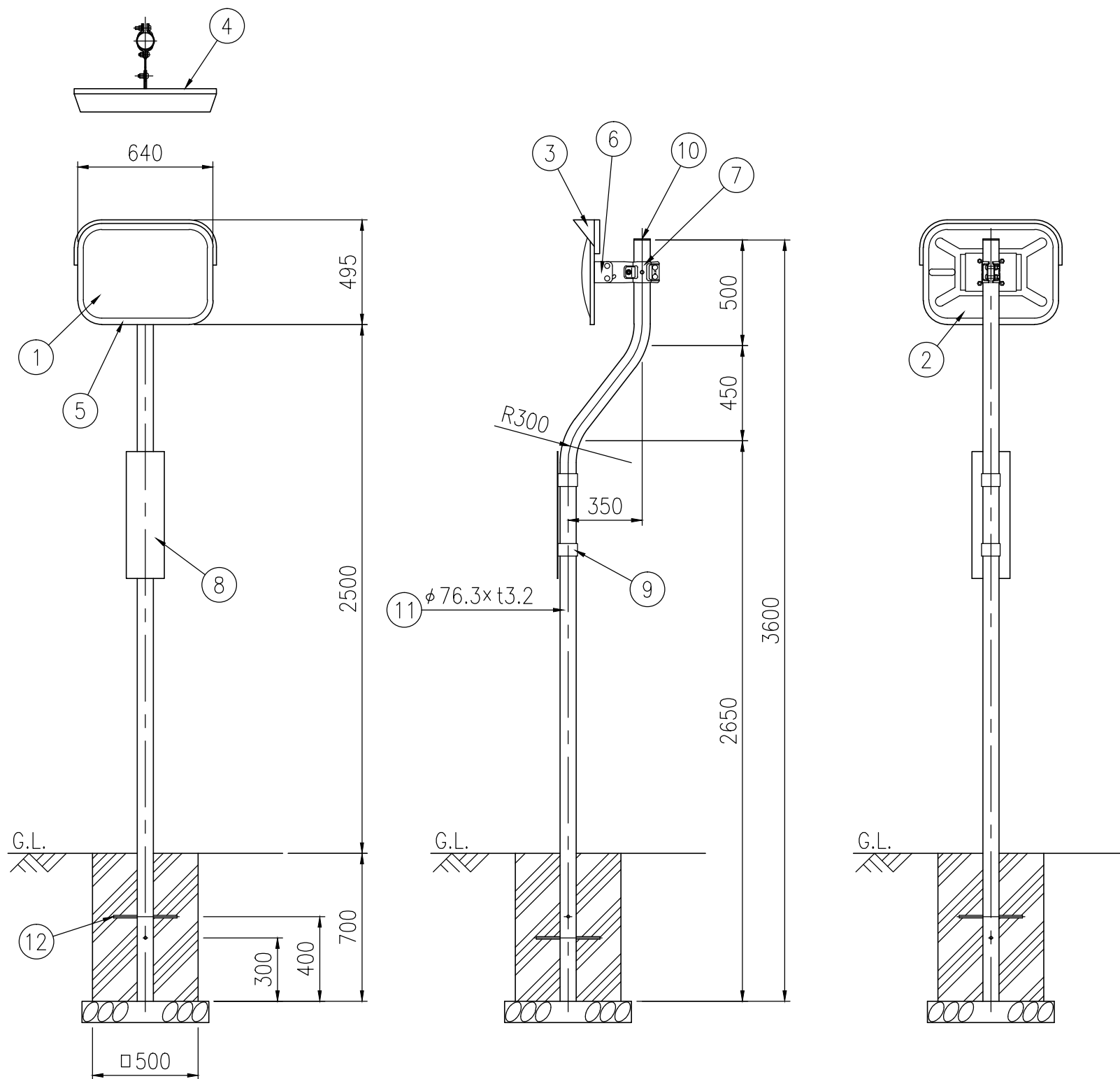
設置図 S=1/25
