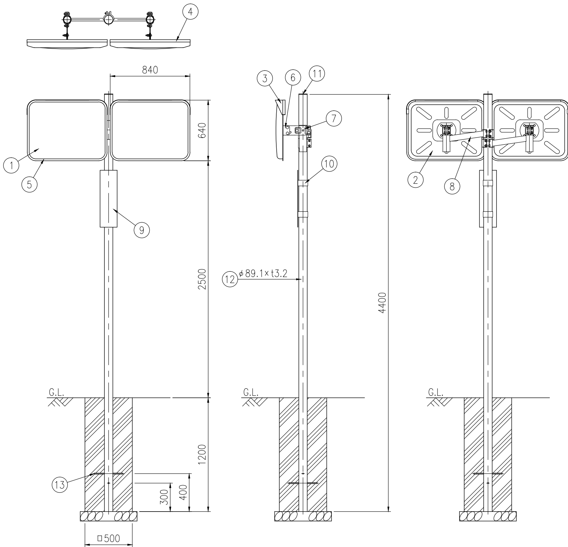
設置図 S=1/25
