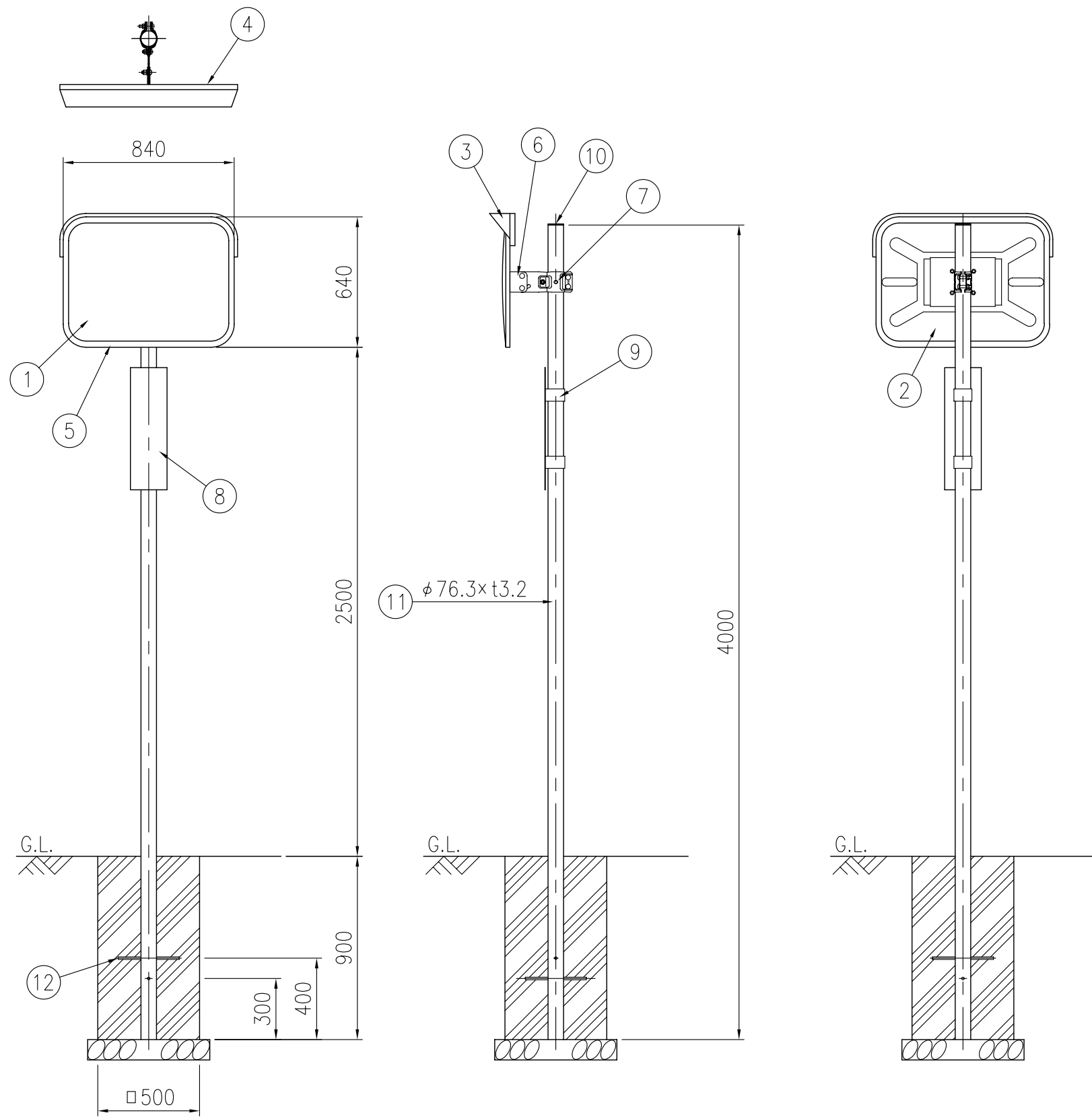
設置図 S=1/25
