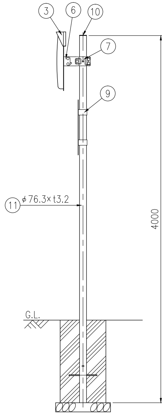
設置図 S=1/25
