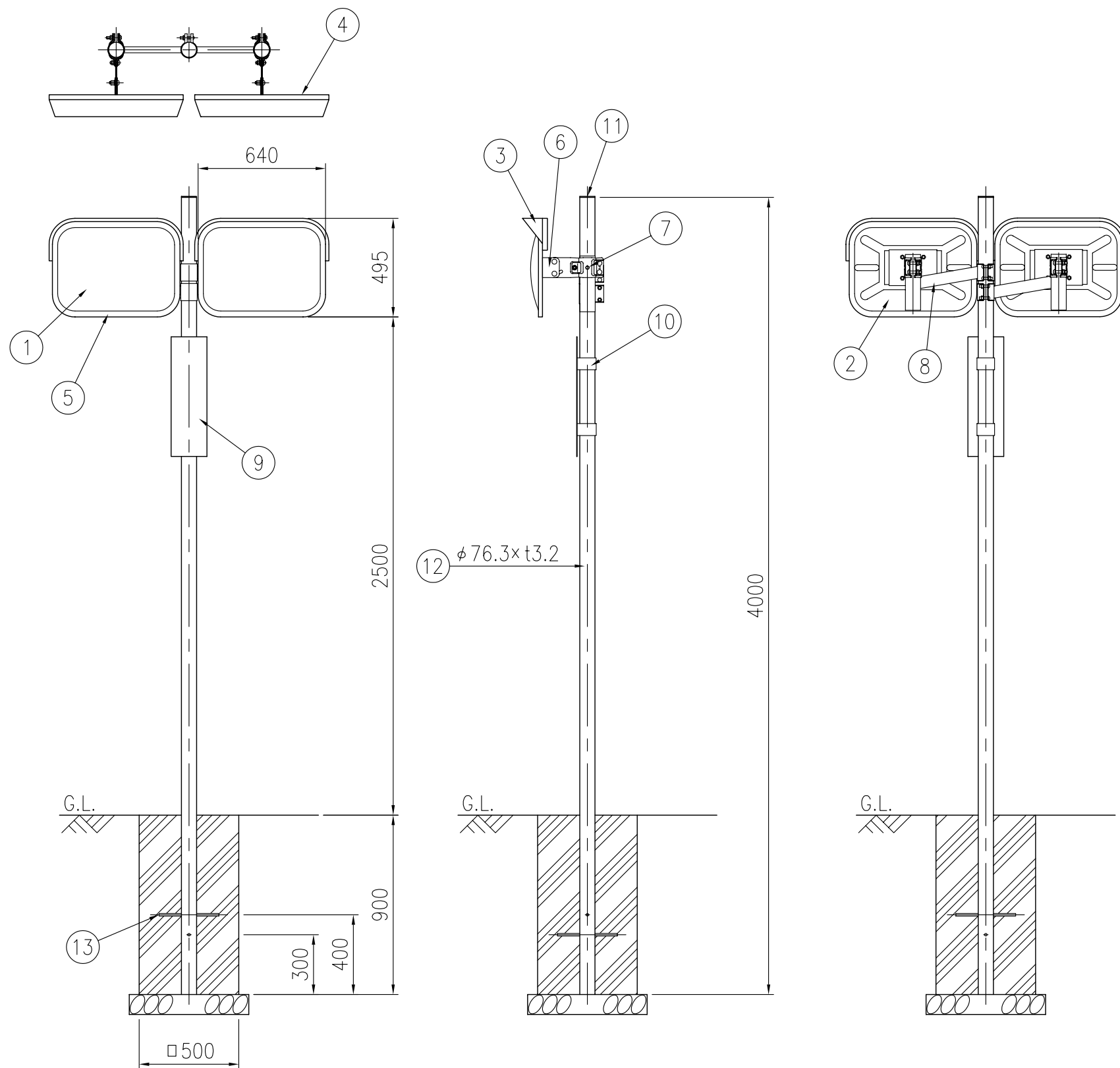
設置図 S=1/25
