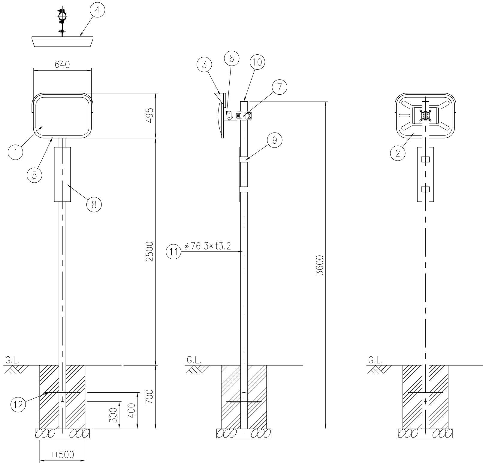
設置図 S=1/25
