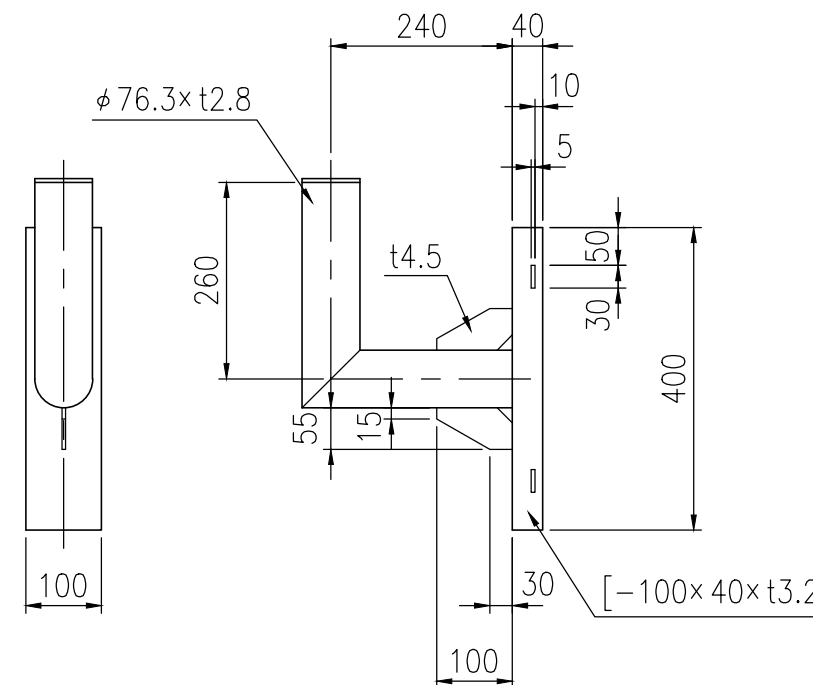
⑦ 電柱取付金具詳細図 S=1/10
