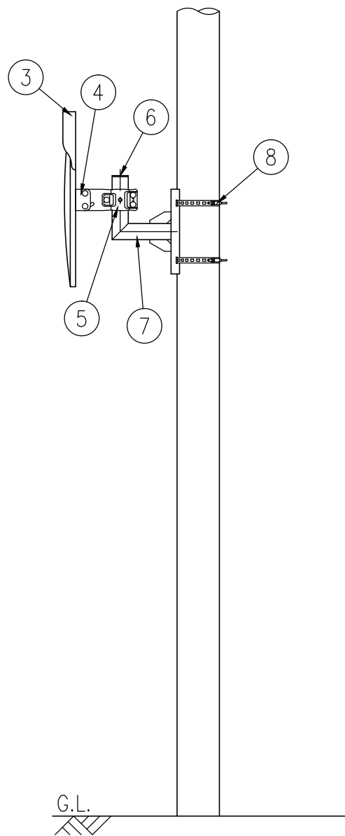
設置図 S=1/25
