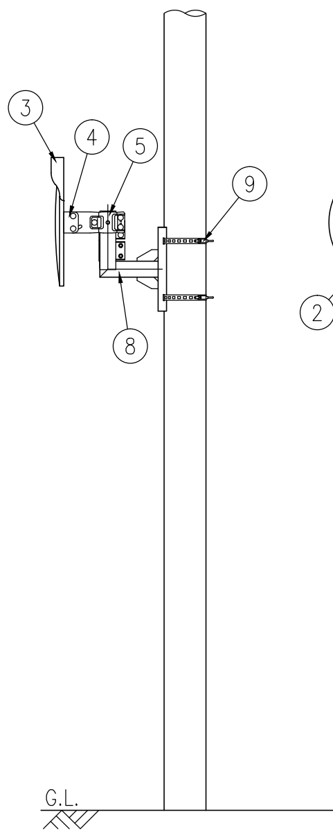
設置図 S=1/25
