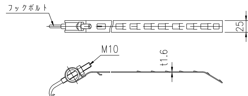
⑧ 取付バンド詳細図 S=1/5
