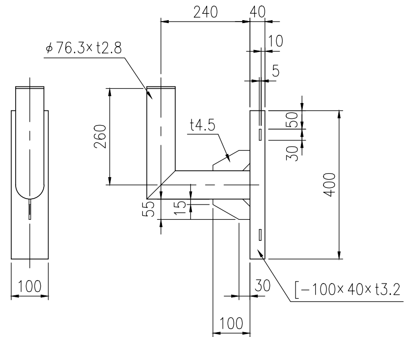
⑦ 電柱取付金具詳細図 S=1/10
