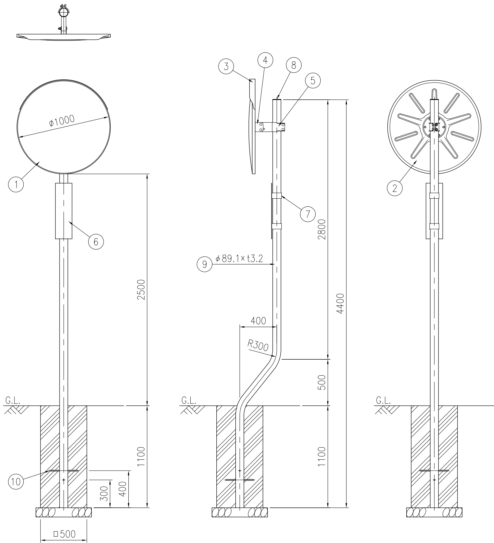
設置図 S=1/25
