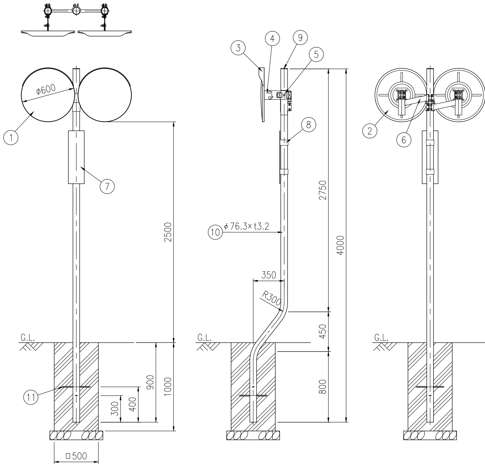
設置図 S=1/25
