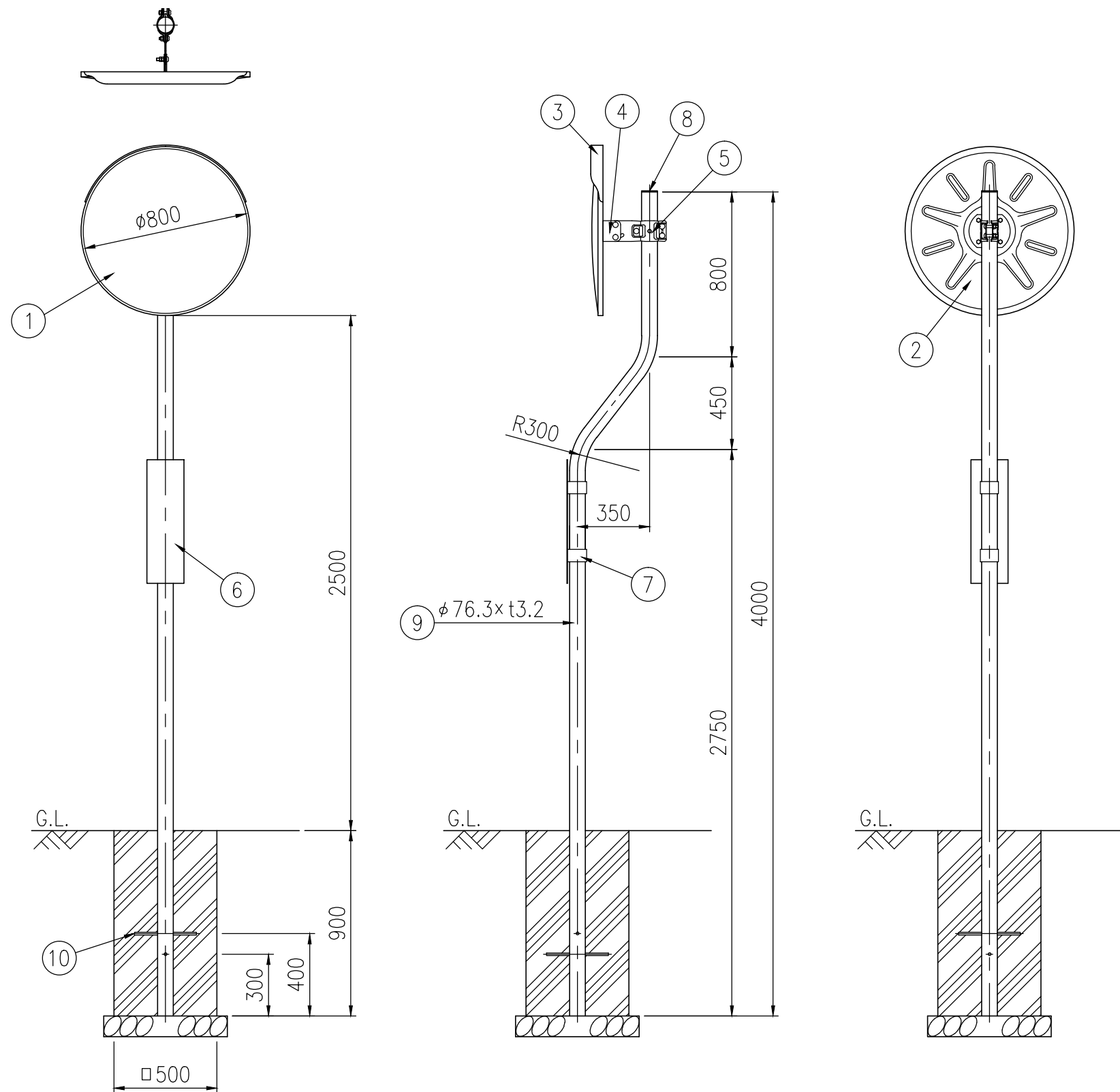
設置図 S=1/25
