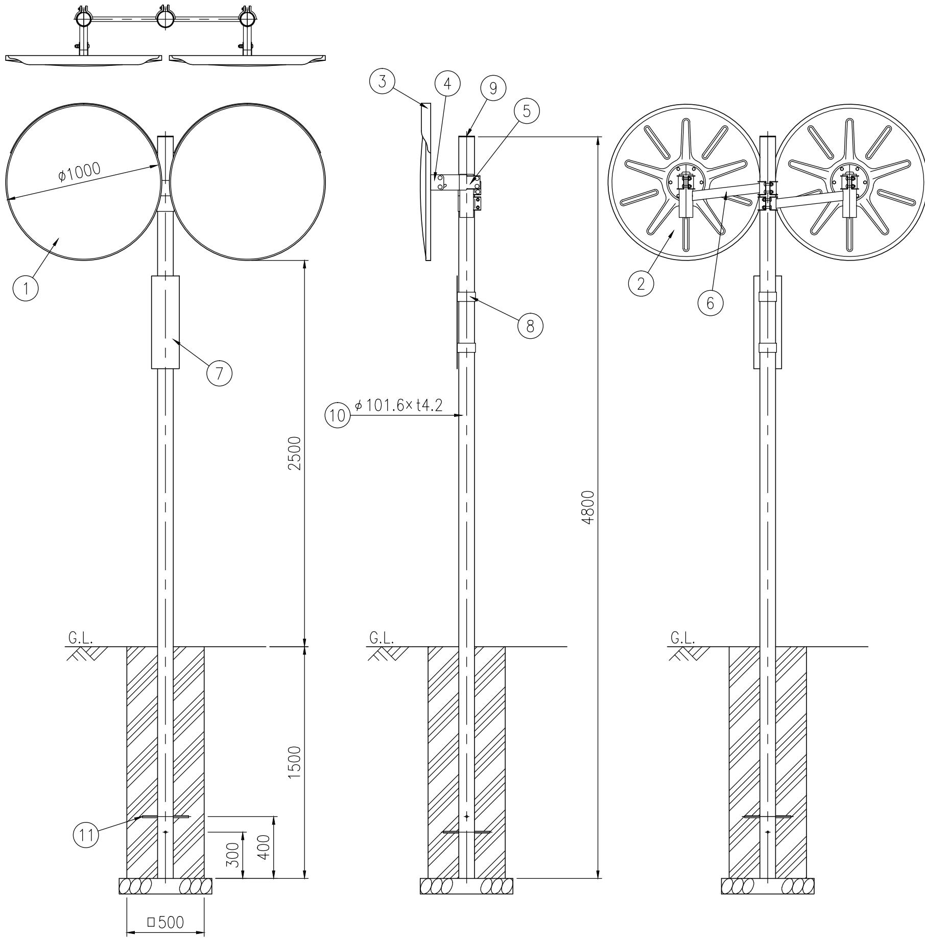
設置図 S=1/25
