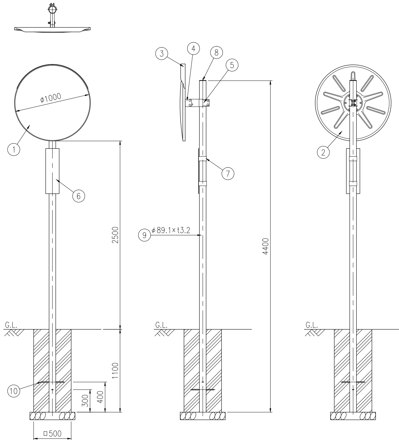
設置図 S=1/25
