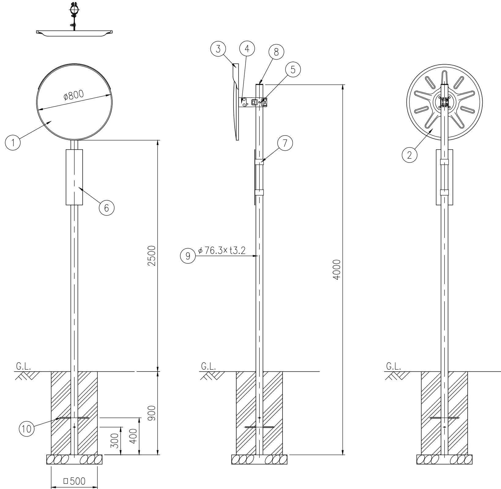
設置図 S=1/25
