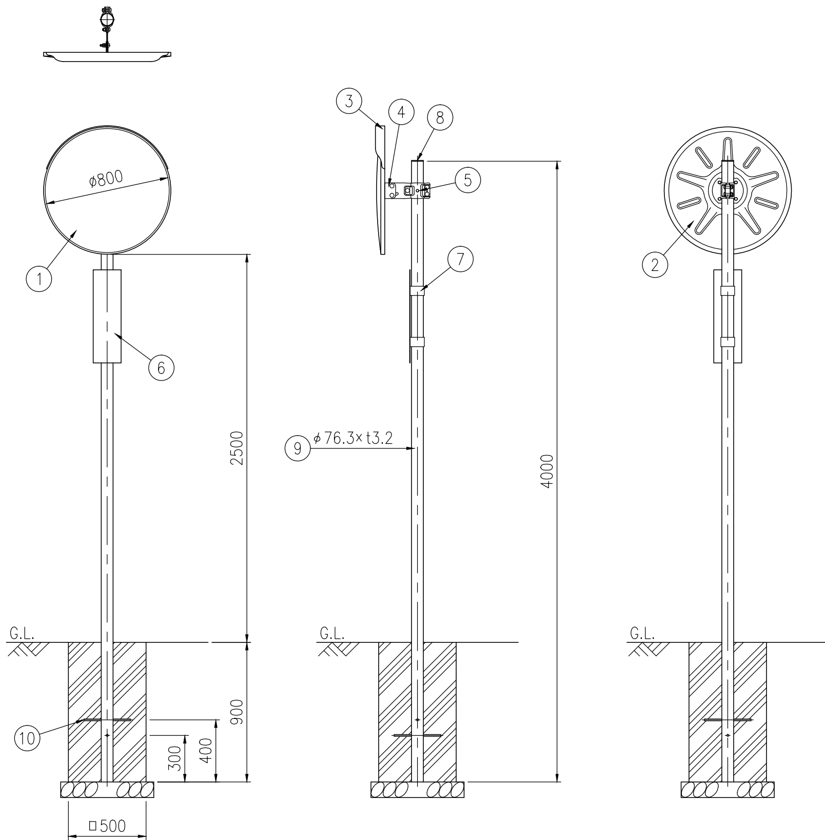
設置図 S=1/25
