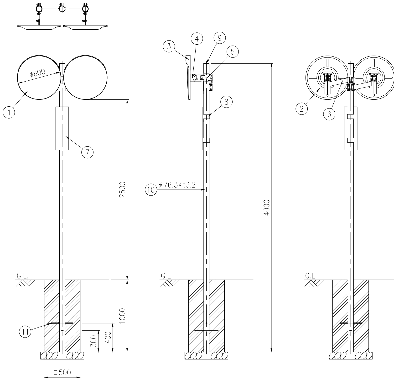
設置図 S=1/25
