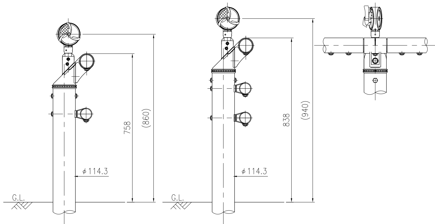
設置図 S=1/10
