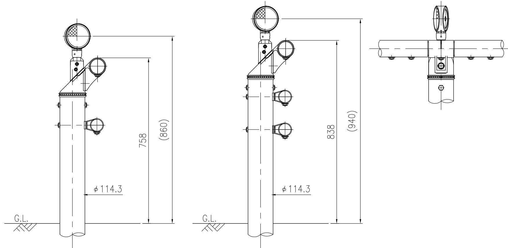
設置図 S=1/10
