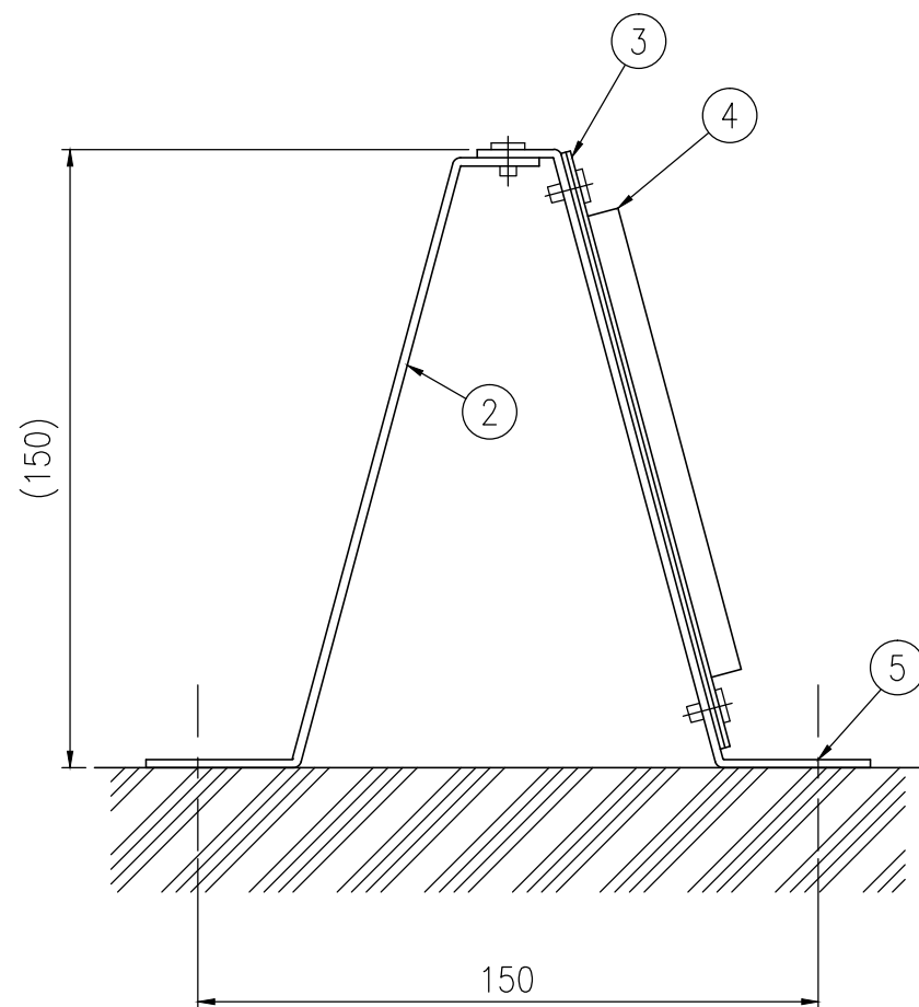
設置図 S=1/10
