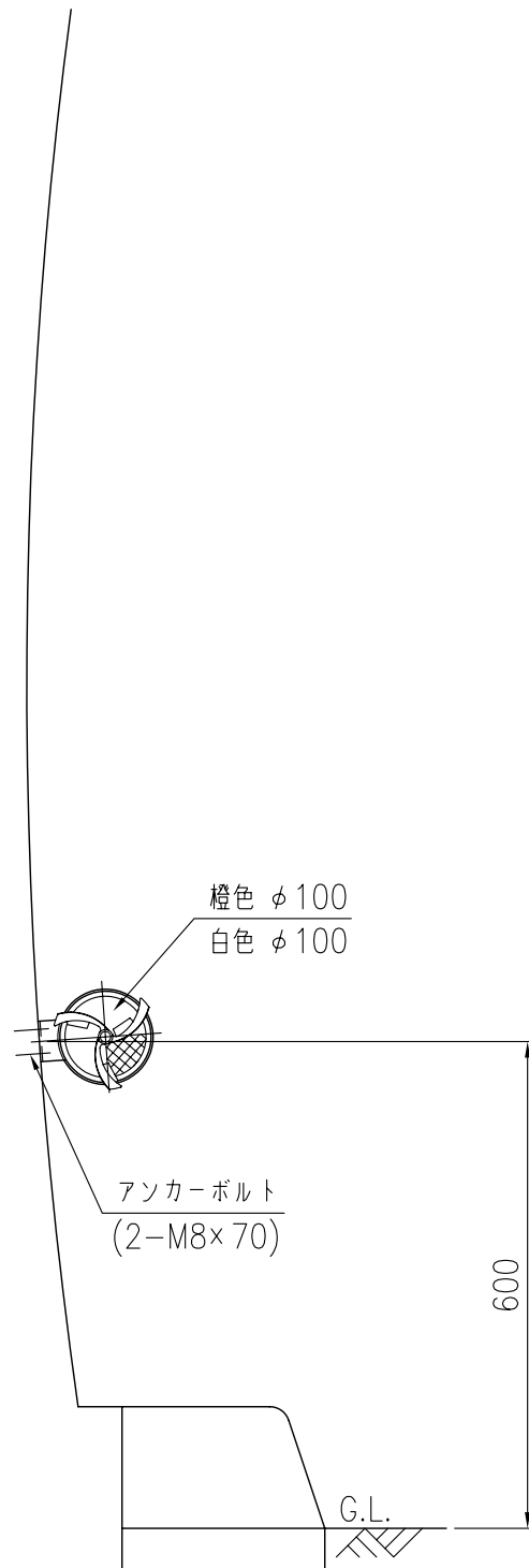
設置図 S=1/10
