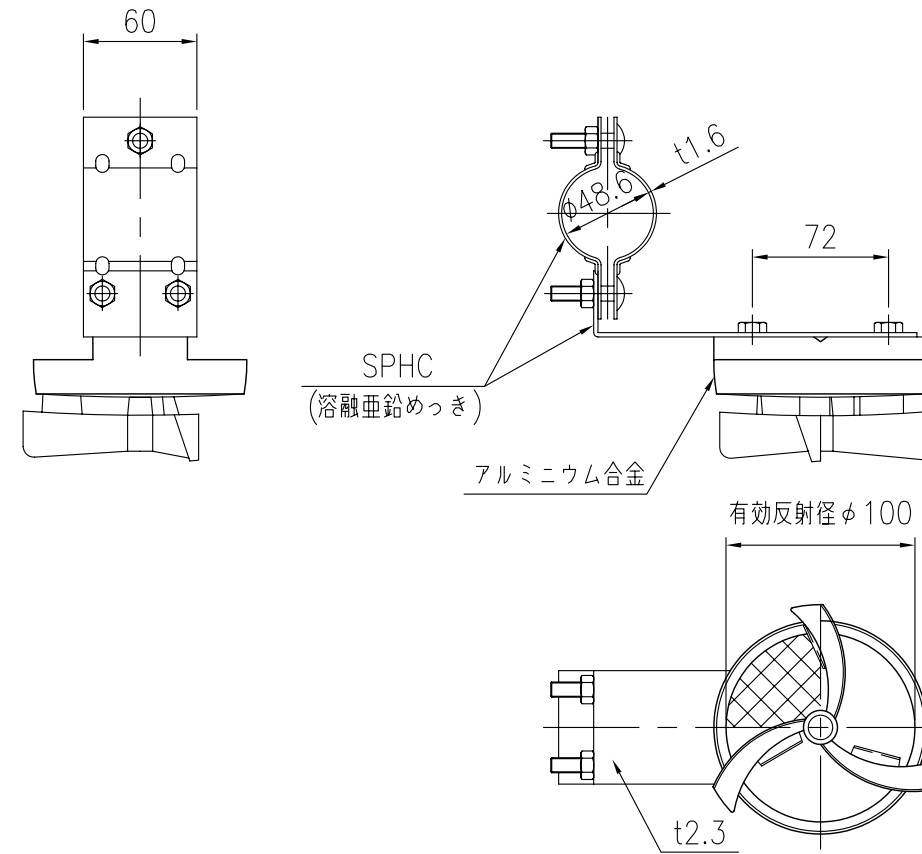
反射部詳細図 S=1/4
