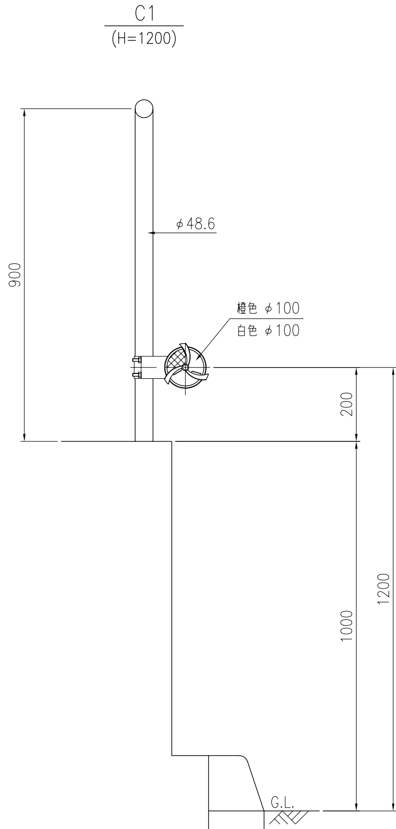
設置図 S=1/10
