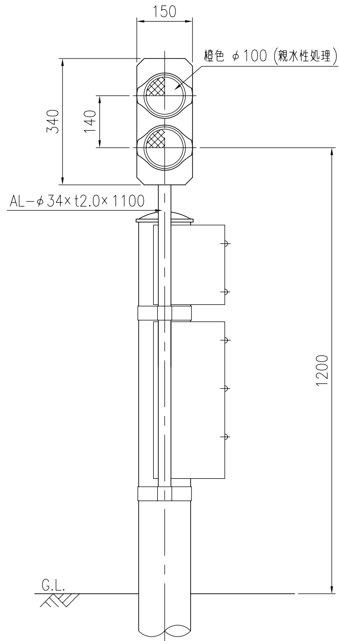
設置図 S=1/10
