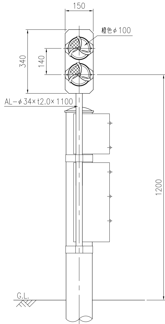
設置図 S=1/10
