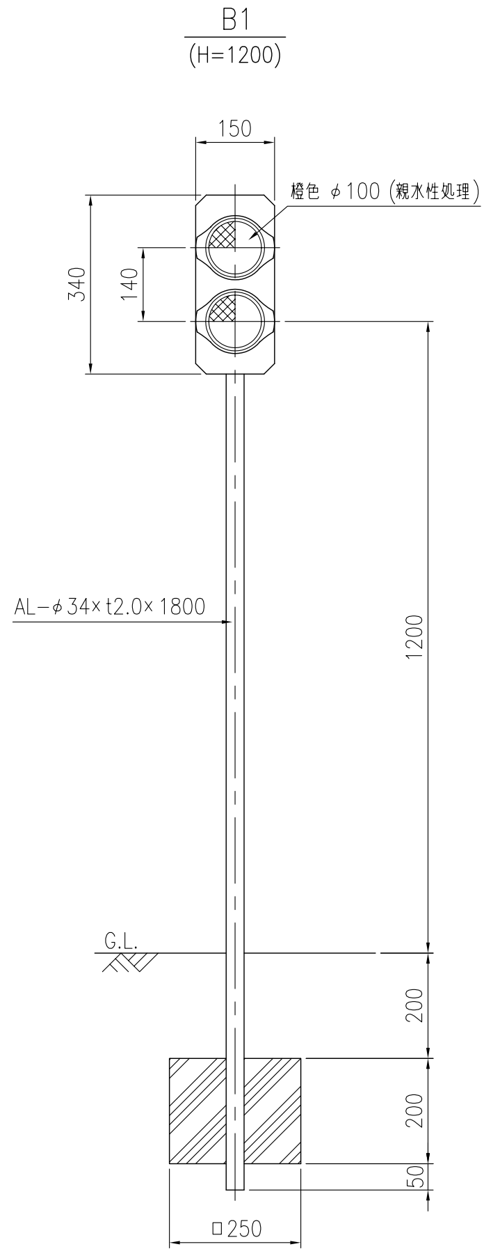
設置図 S=1/10
