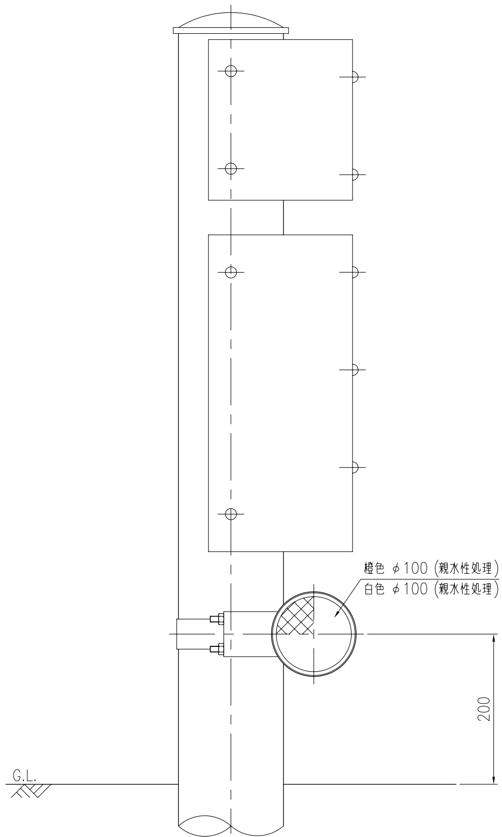
設置図 S=1/5
