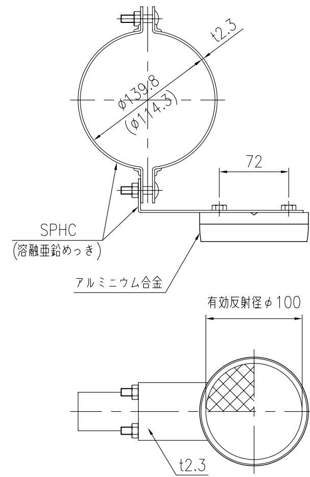
反射部詳細図 S=1/4
