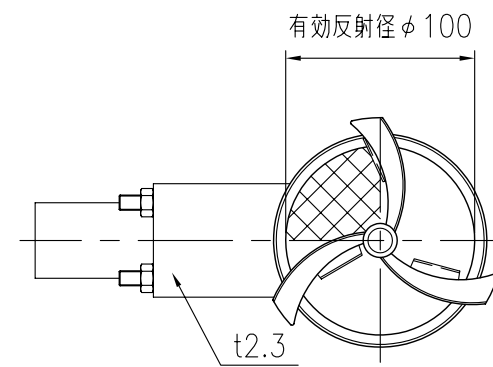
反射部詳細図 S=1/4
