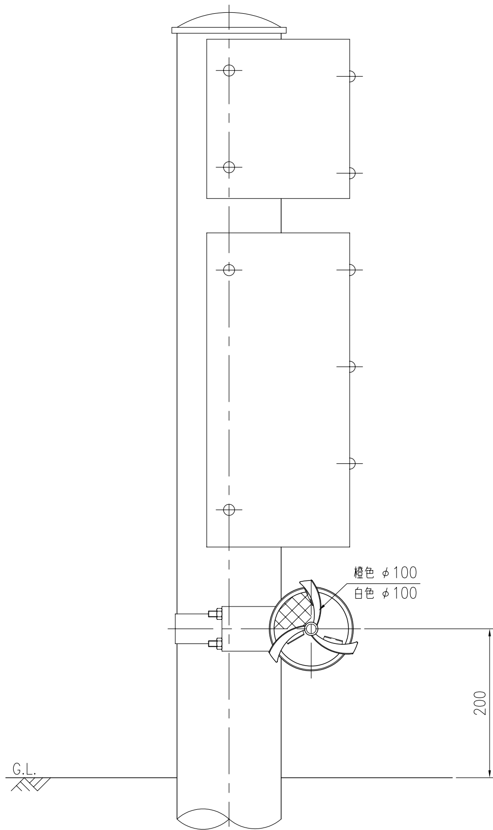
設置図 S=1/5
