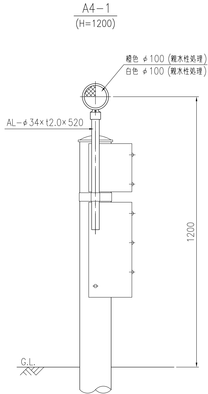
設置図 S=1/10
