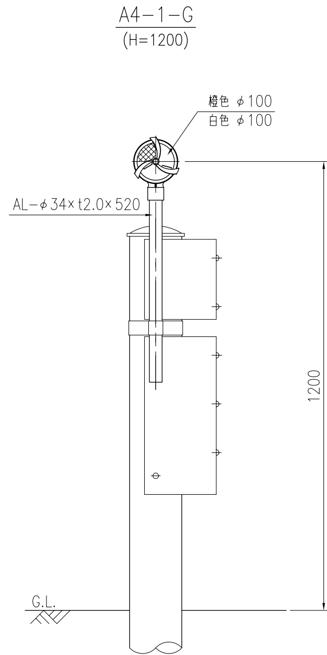
設置図 S=1/10
