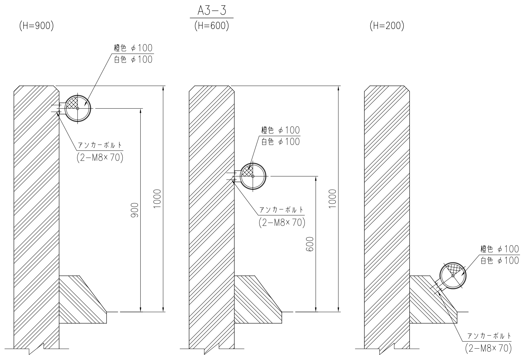
設置図 S=1/10
