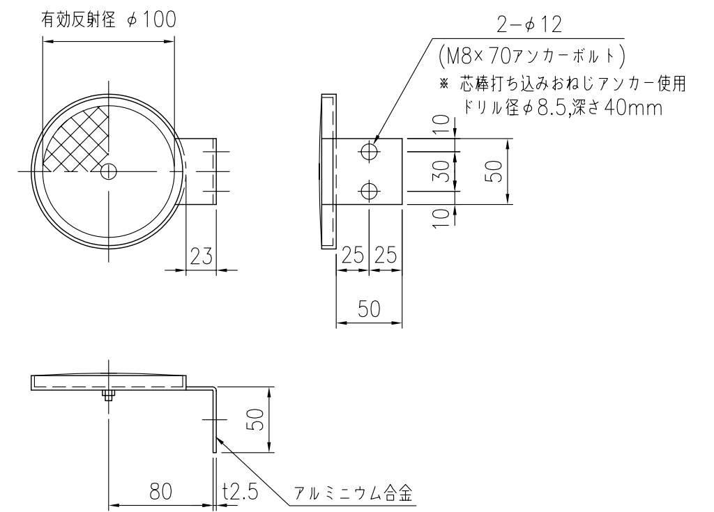
反射部詳細図 S=1/4
