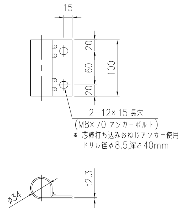
よう壁取付金具詳細図 S=1/4
