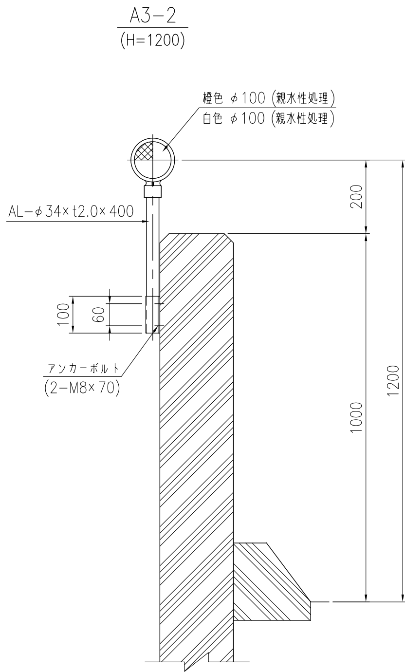
設置図 S=1/10
