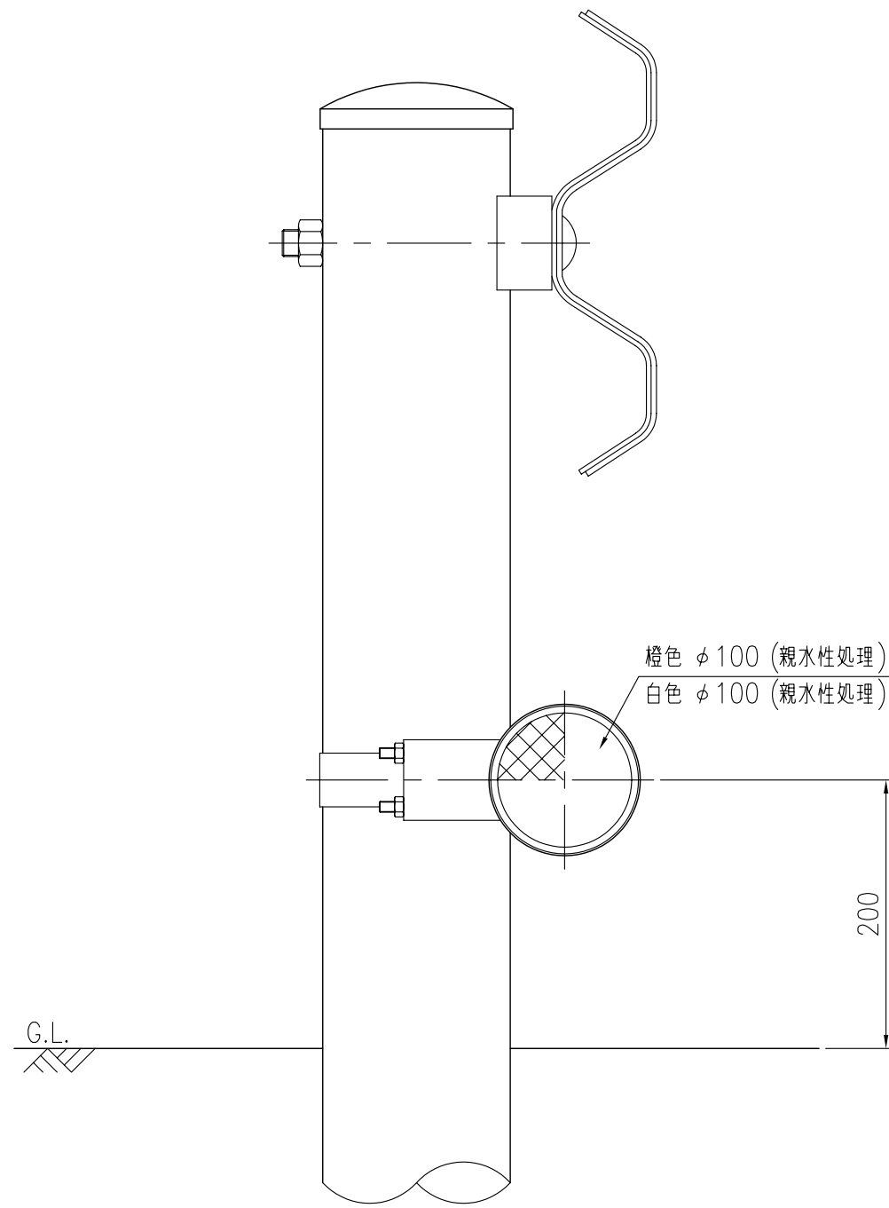
設置図 S=1/5
