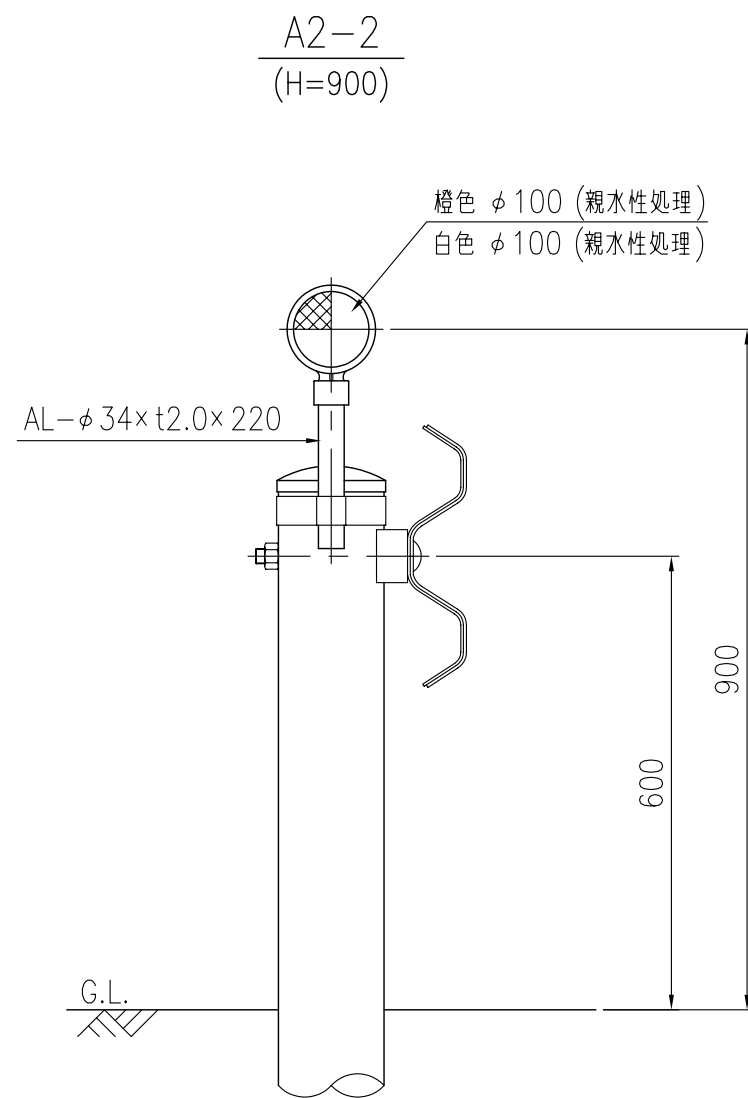
設置図 S=1/10
