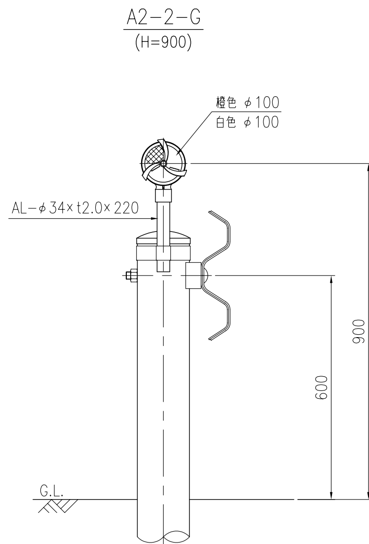
設置図 S=1/10
