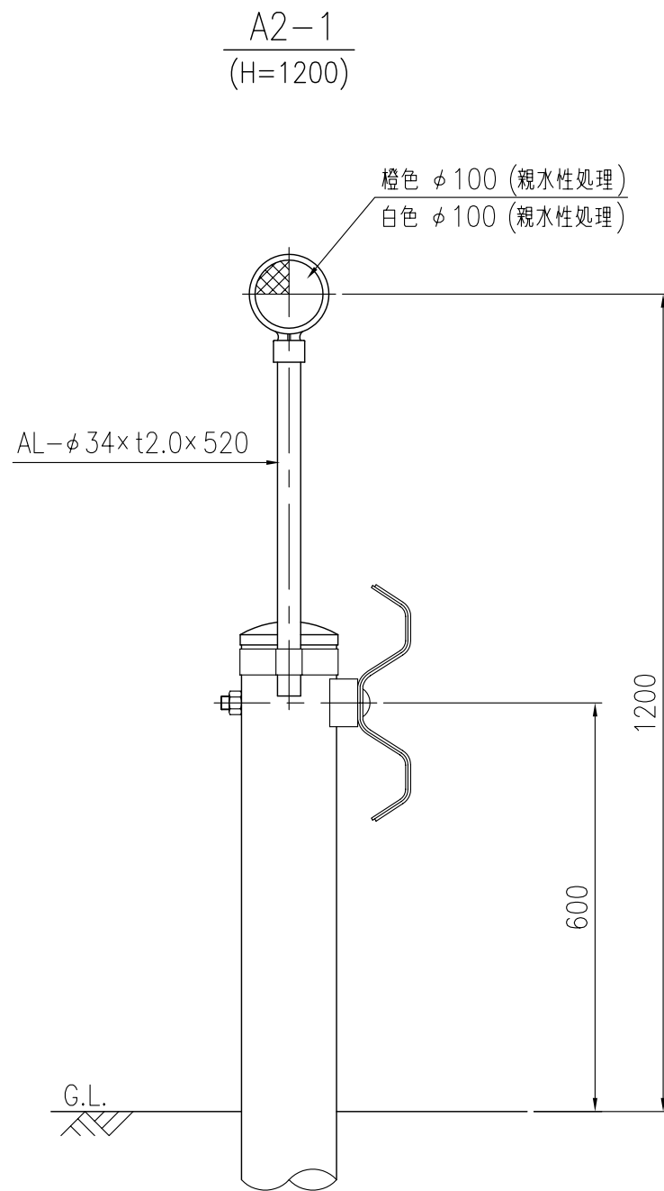
設置図 S=1/10
