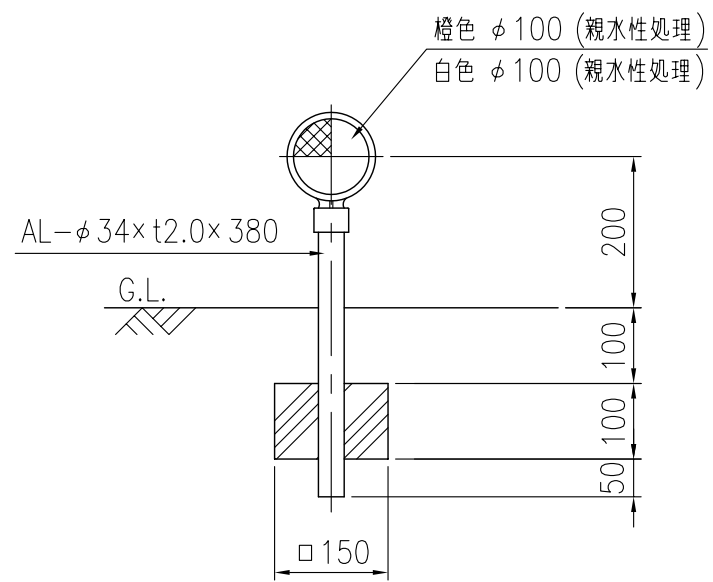
設置図 S=1/10
