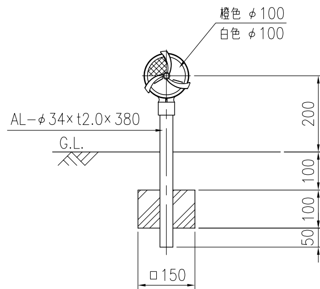
設置図 S=1/10
