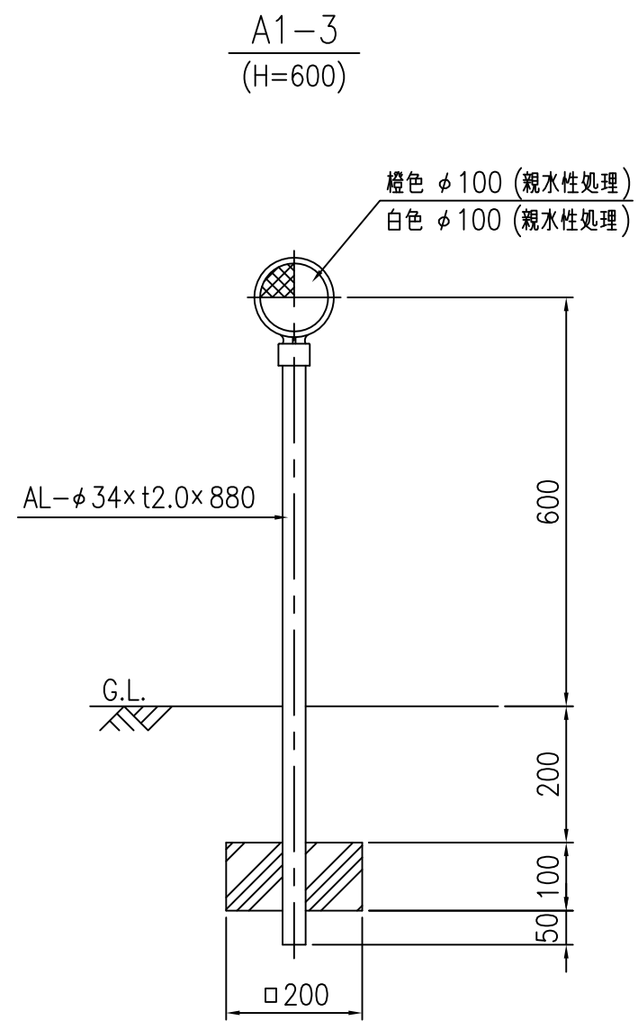
設置図 S=1/10
