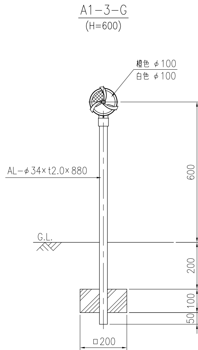
設置図 S=1/10
