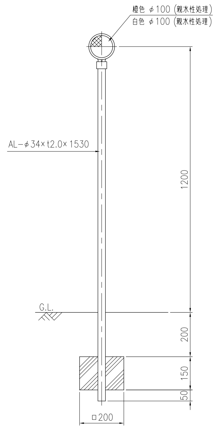
設置図 S=1/10
